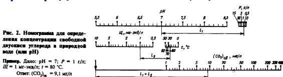
"Рис.2. Номограмма для определения концентрации свободной двуокиси углерода в природной воде (или pH)"
