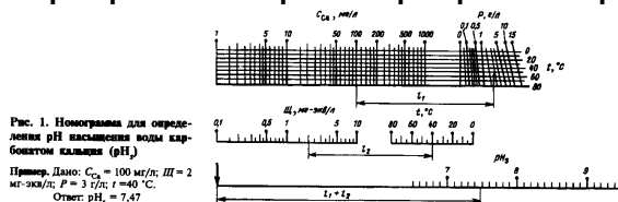
"Рис. 1. Номограмма для определения pH насыщения воды карбонатом кальция (pH s )"
