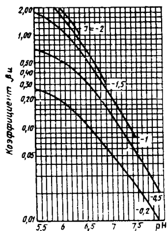
Рис. 4. Номограмма для определения коэффициента \beta при расчете дозы щелочи
